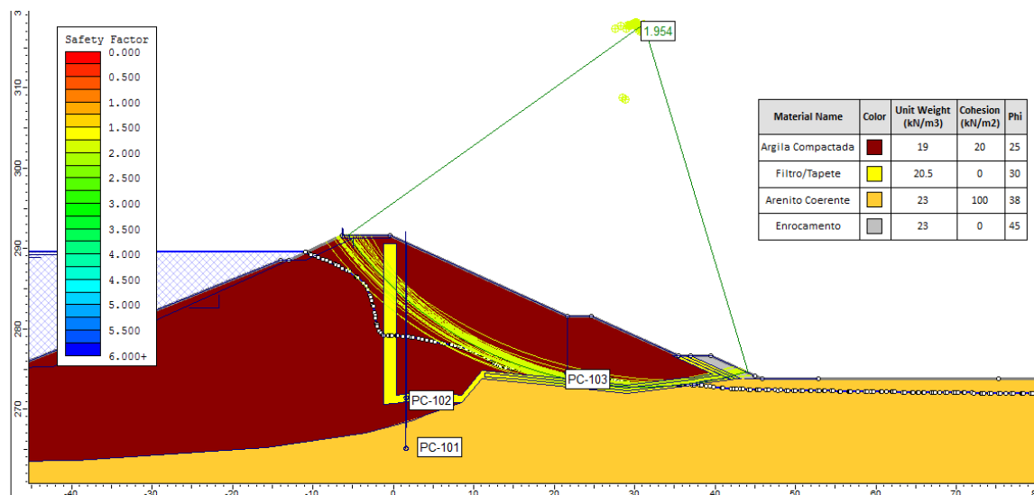
Figura 11 - Seção 4+00,00 – Resultado da análise de estabilidade considerando a instrumentação - Fator de Segurança igual a 1,95
