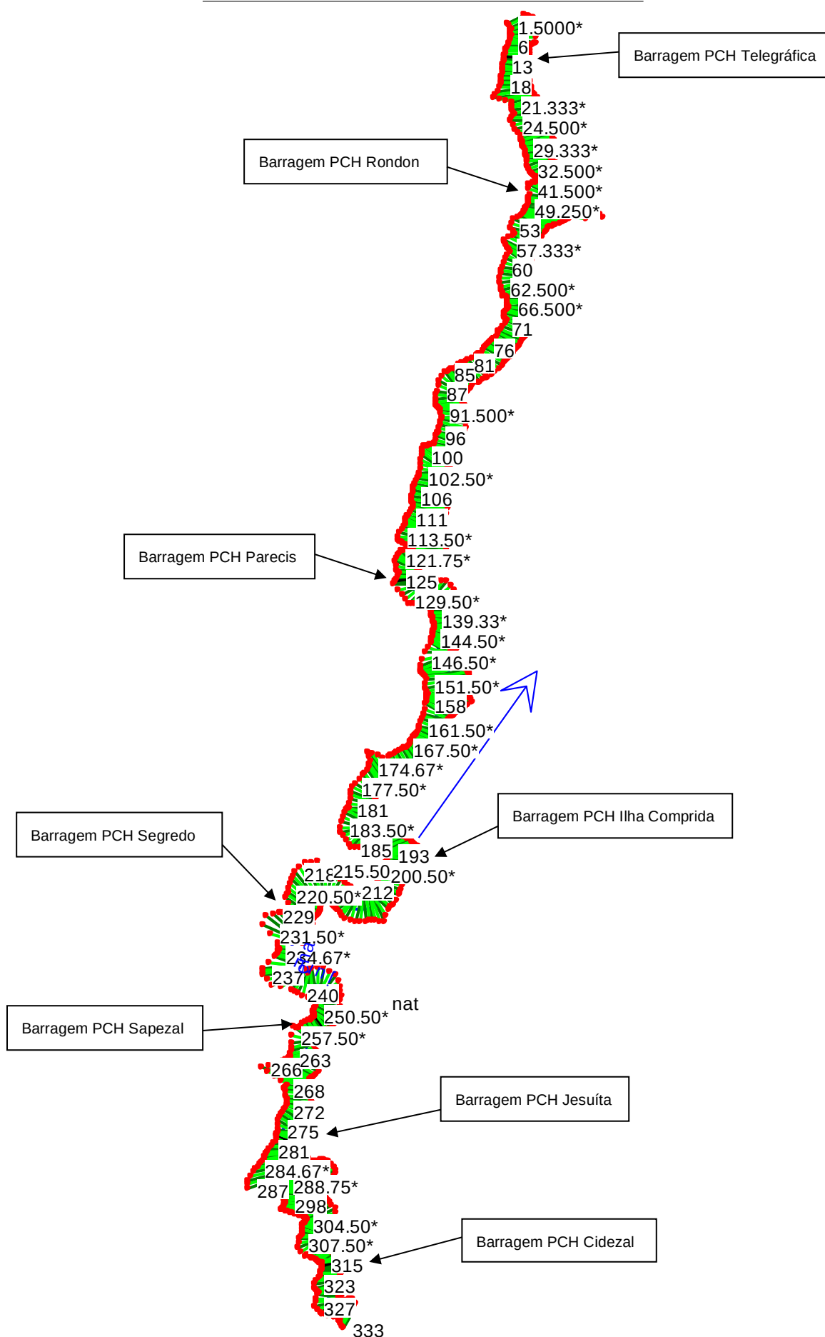
Figura 21 – Seções lançadas no Hec-Ras
