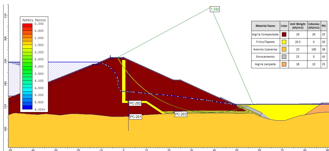
Figura 12 - Seção 6+10,00 – Resultado da análise de estabilidade considerando a instrumentação - Fator de Segurança igual a 1,59
