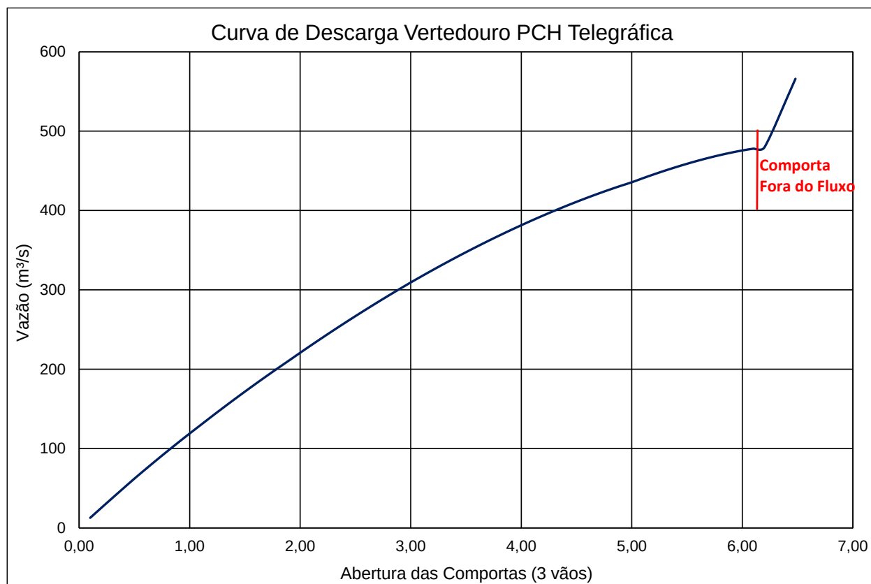
Gráfico 5 – Curva de Descarga Vertedouro – PCH Telegráfica
