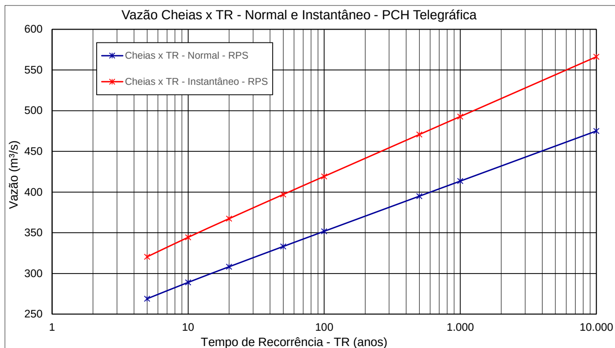
Gráfico 1 – Vazão e Tempo de Recorrência
