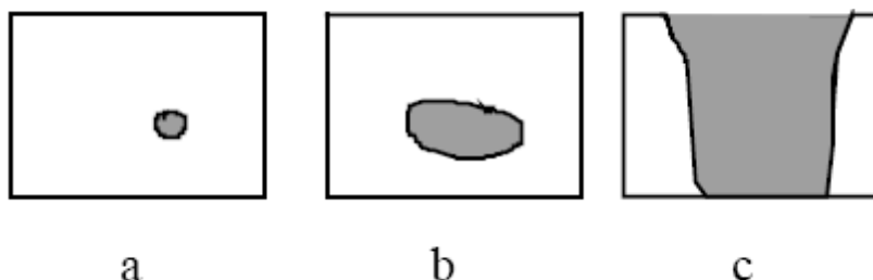
Figura 15 – Formação da brecha por infiltração
