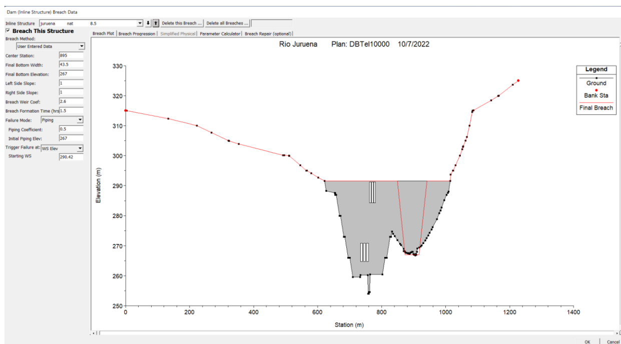
Figura 23 – Dados do Barramento terra – Hec-Ras
