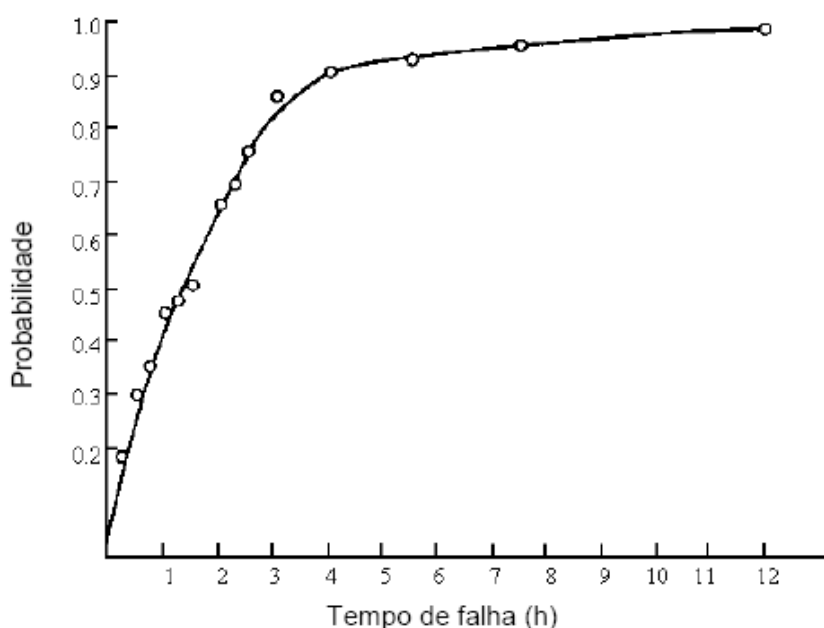
Figura 18 – Tempo de formação da brecha
