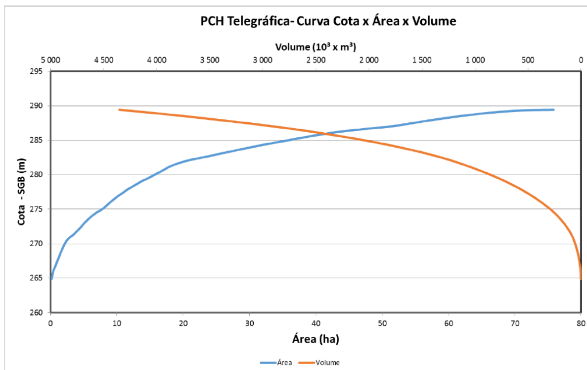
Figura 6 – PCH Telegráfica – Curva CAV
