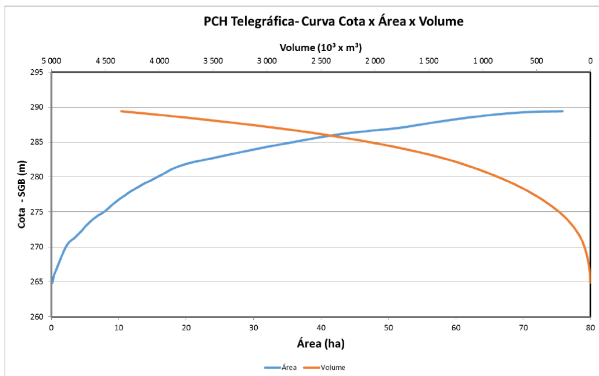
Figura 20 – PCH Telegráfica – Curva CAV
