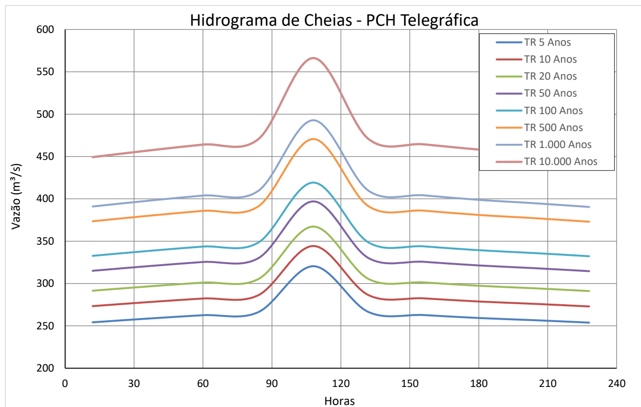
Gráfico 4 – Hidrograma de cheias PCH Telegráfica
