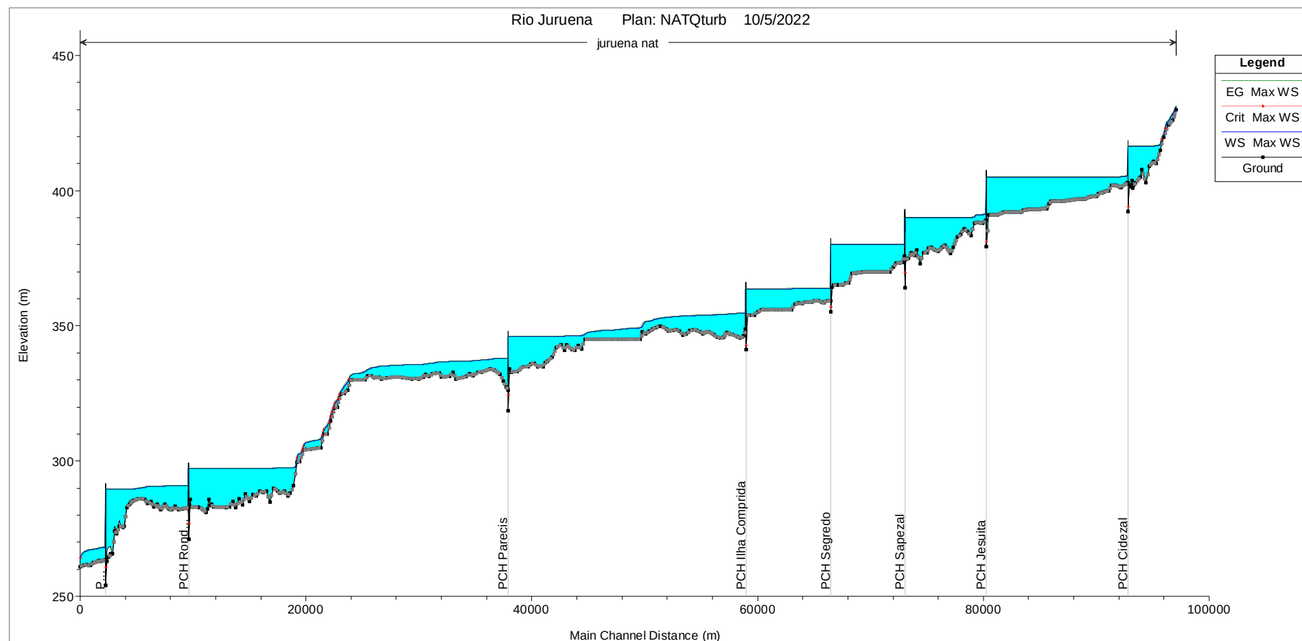
Figura 22 – Perfil do Rio Juruena com Barramento com Dia de Sol - Qturb
