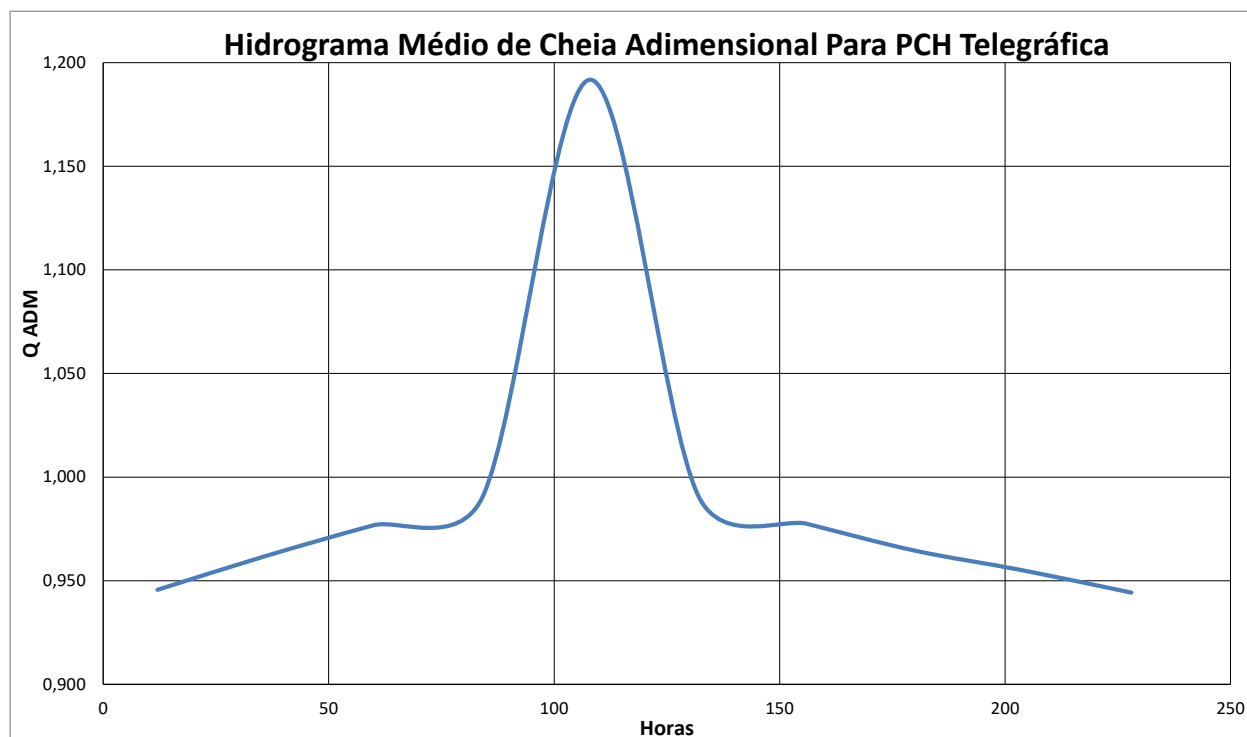
Gráfico 3 – Hidrograma Médio Cheia adimensional PCH Telegráfica
