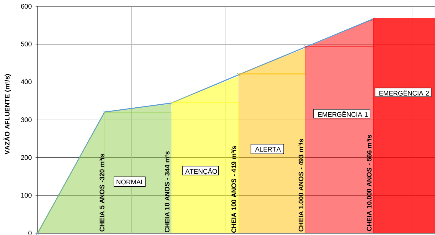
PCH TELEGRÁFICA - CURVA REFERENCIAL DA BARRAGEM
